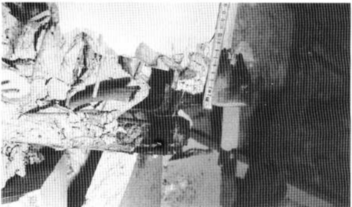
KUVA 2. Poikkileikattu oikeanpuoleinen U-palkki, jossa näkyy puu-tuen saumakohta.
